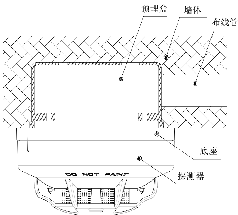
图3 JTF-GOM-TX3120 安装示意图
