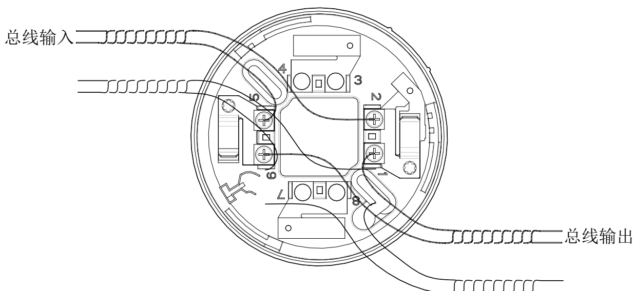
图 4 JTF-GOM-TX3120 接线方式
