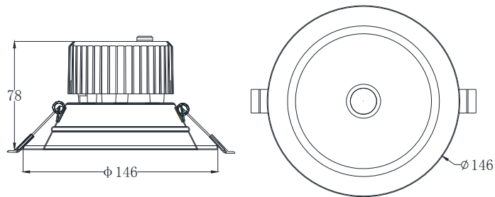
图 4.2 灯具外形尺寸，单位 mm (TS6630G\ TS6631G)
