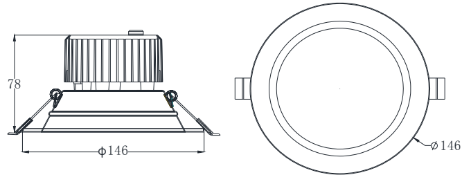
图 4.1 灯具外形尺寸，单位 mm (TS6630\ TS6631)
