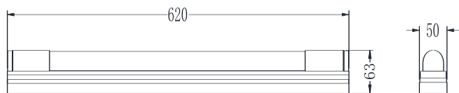
图 4.1 灯具外形尺寸，单位 mm（TS-ZFJC-E9W-6620A）
