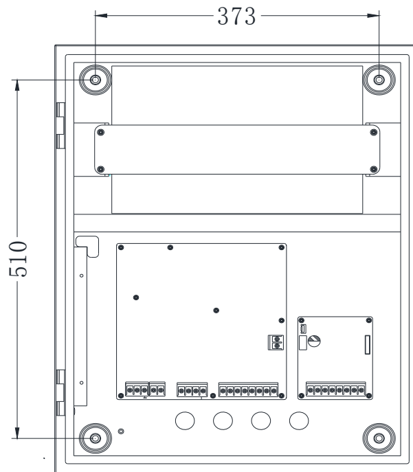
图 2 内部结构及安装尺寸图
