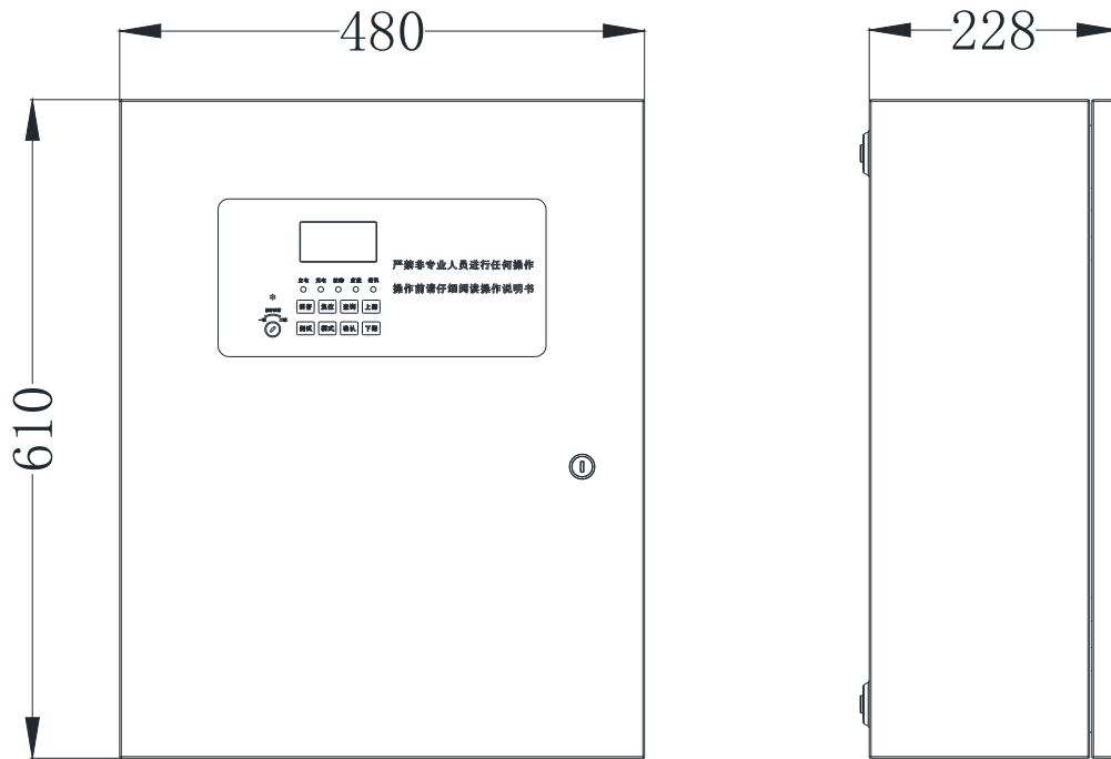
图 1 外观尺寸图
