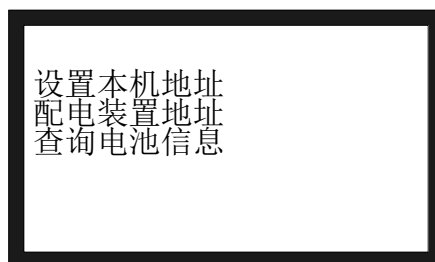
图 5 设置界面
