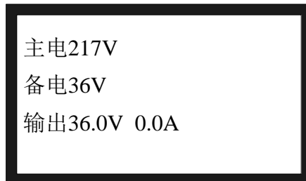
图 4 监控界面
