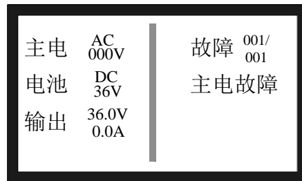
图 8 故障界面
