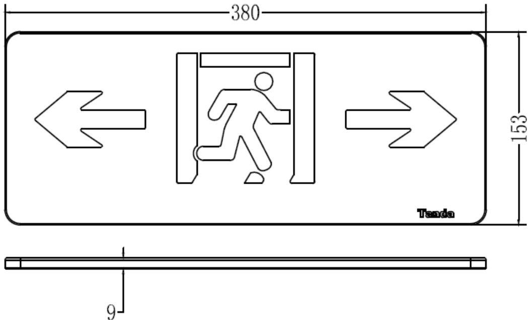
图 1 壁挂式标志灯具外形尺寸
