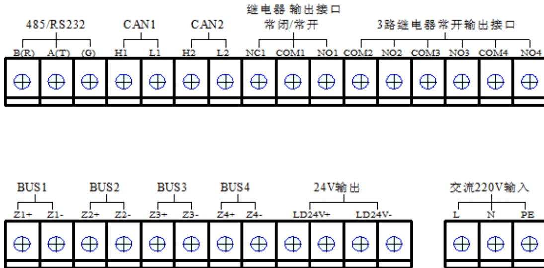
图 4-4 控制器外接端子
