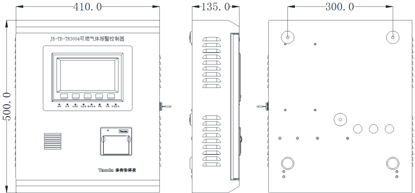
图 4-1 产品尺寸图
