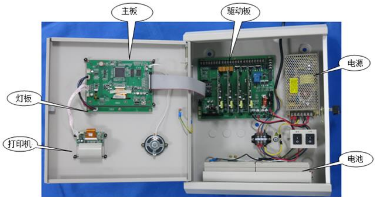
图 4-3 控制器内部结构说明
