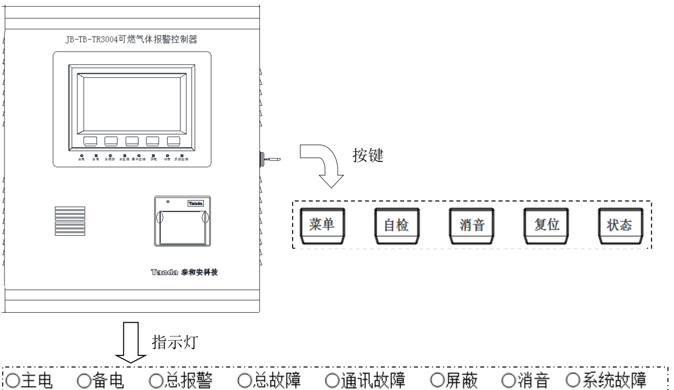
图 4-2 按键与指示灯
