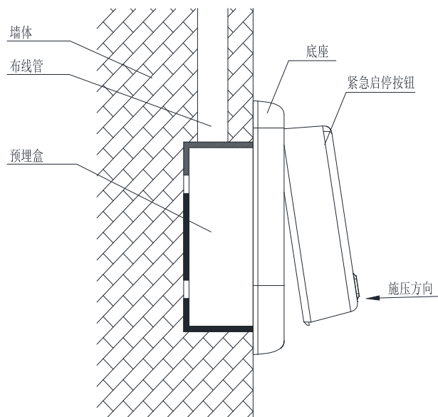
图 3 安装示意图
