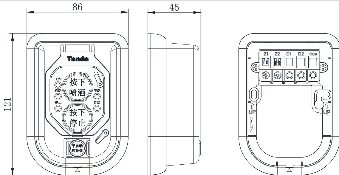
图 1 产品及底座外形示意图
