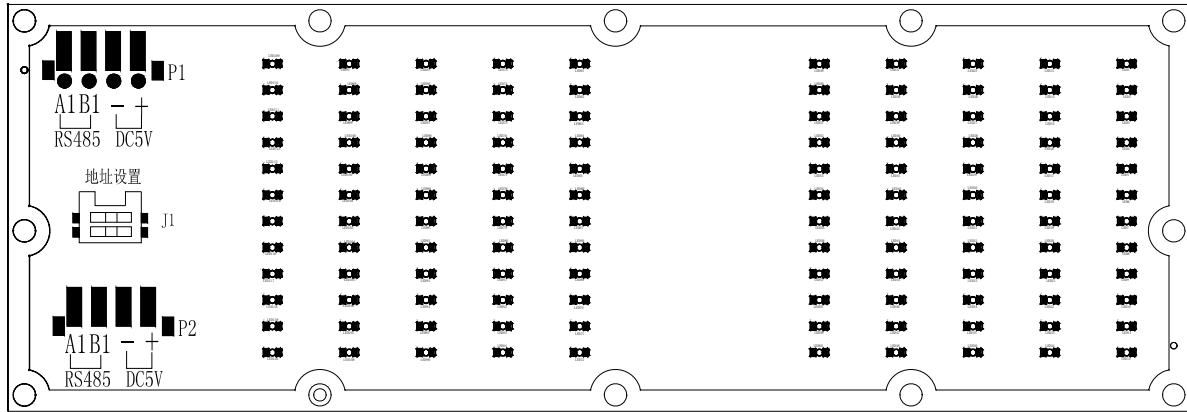
TG3400广播分配盘背面示意图
