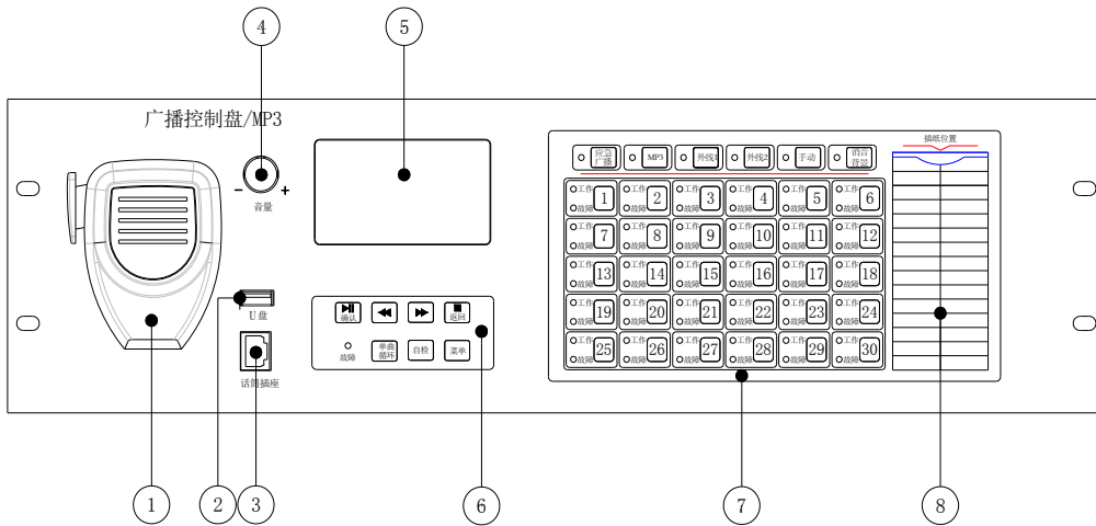
前面板功能图
