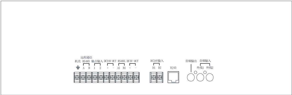
后面板接线端子图
