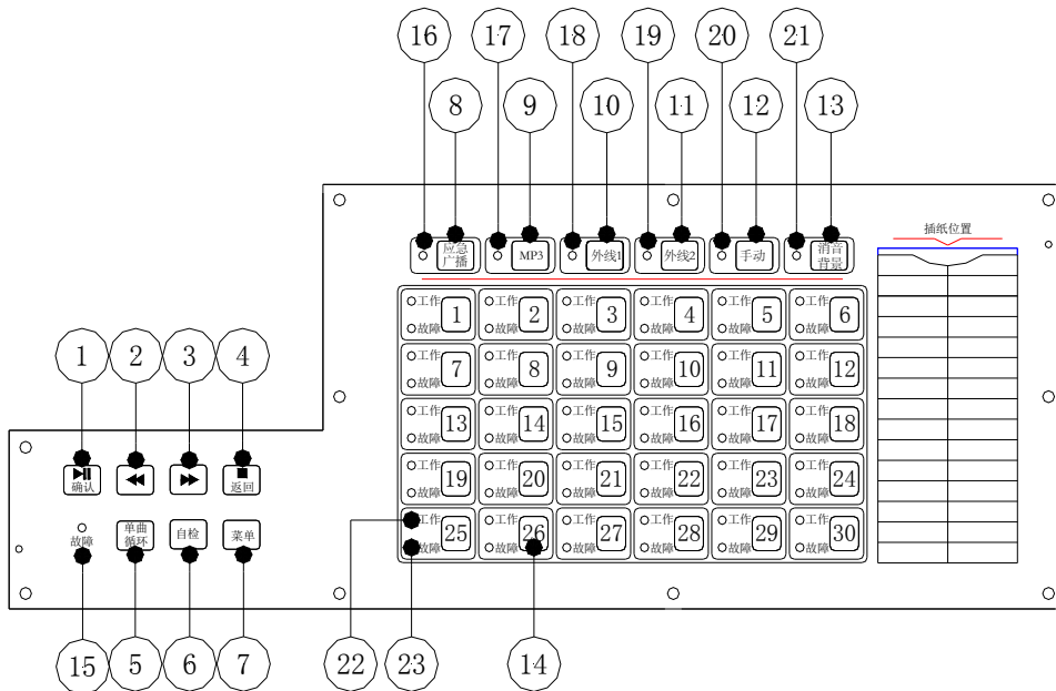
指示灯/按键详细说明图
