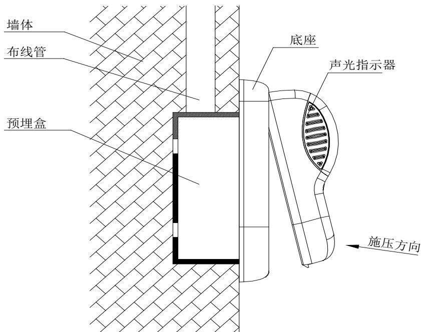
图2 安装示意图
