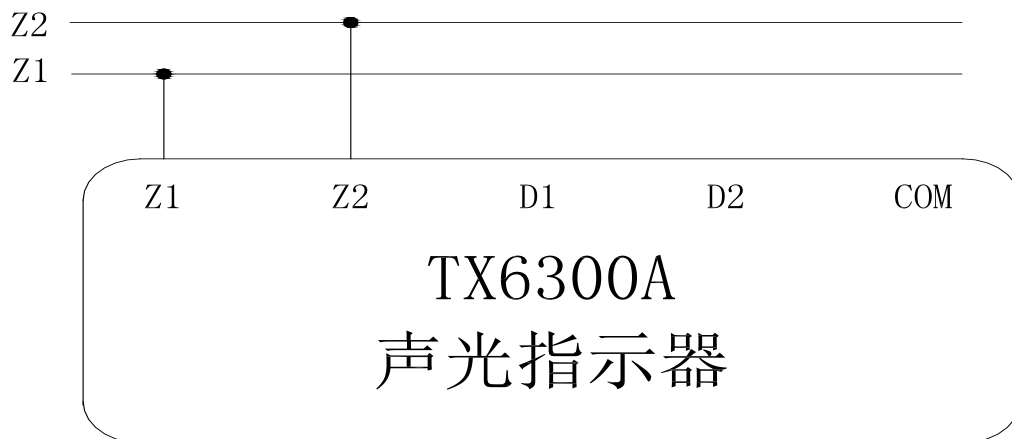
图 3 接线方式示意图
