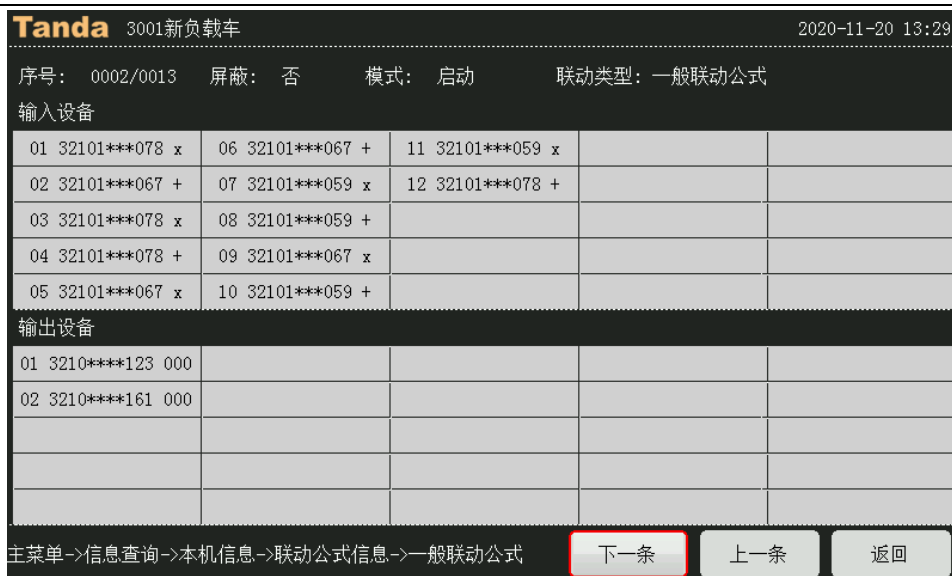
图 4-10 联动公式信息界面
