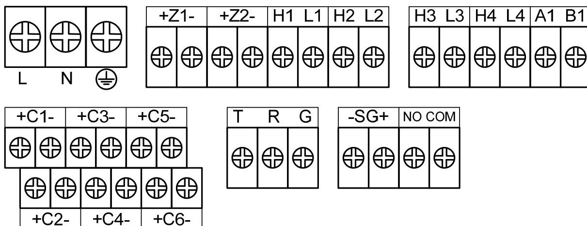
图 5-2 控制器对外接线端子示意图
