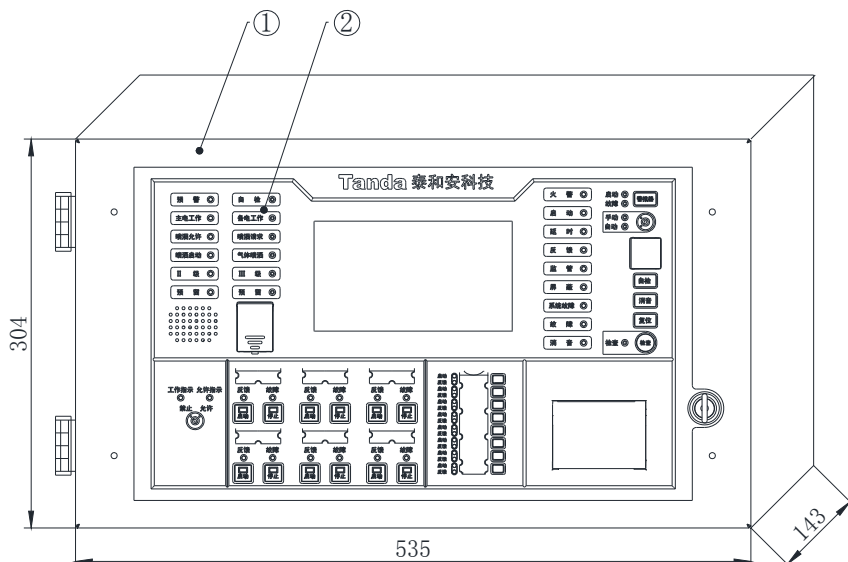
图 2-1 控制器外观结构示意图
