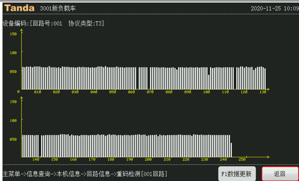
图 4-8 重码检测界面
