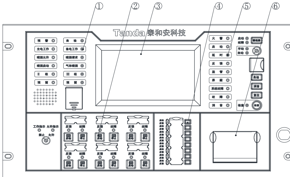
图 2-2 主面板示意图
