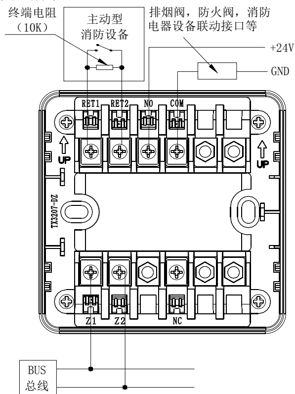
图 3 接线方式示意图
