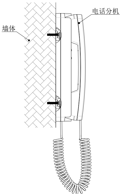
图 2：安装示意图
