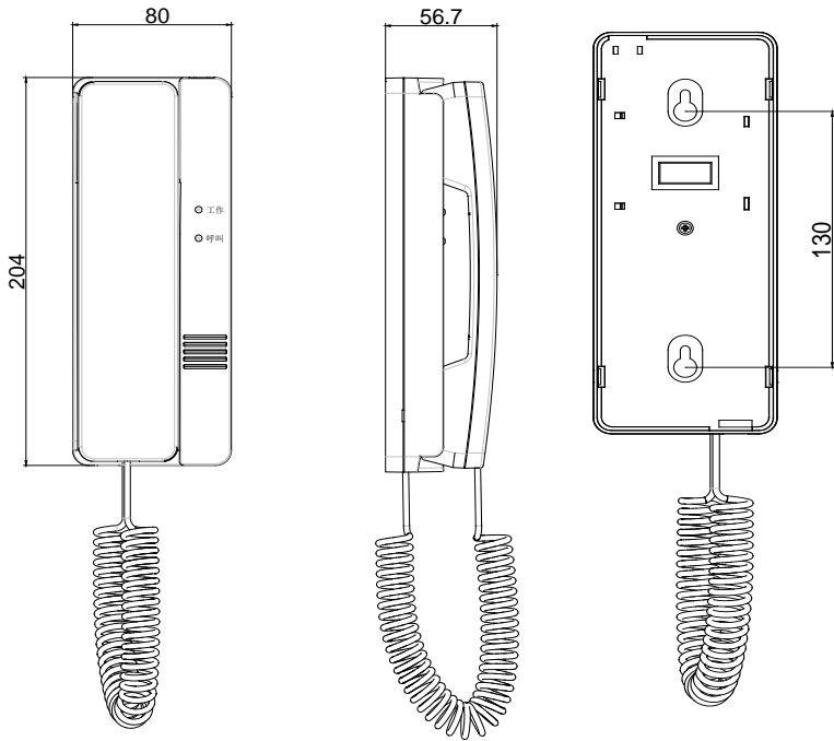
图 1 外形尺寸及安装示意图
